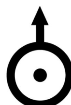
Uranus
