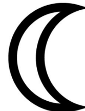
Moon
