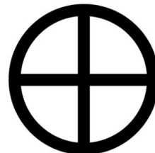
Earth
