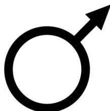
Mars
